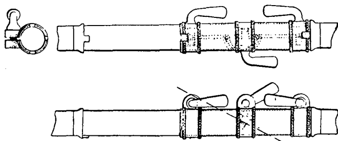
FIG. 5. — BICYCLETTE PLIANTE. — Le manchon et son système de serrage.
