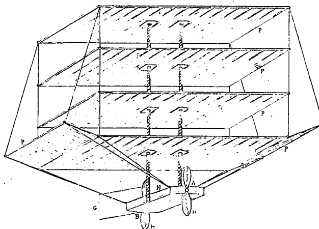
Aéroplane vu par dessous.
