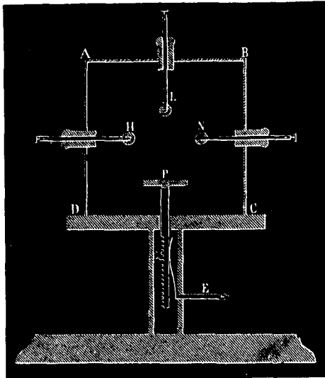
Figure 93. — Appareil de Ducretet.
