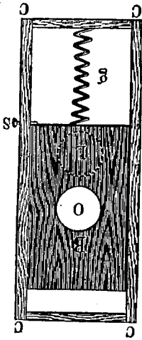
Figure 9. Obturateur dit à guillotine.
