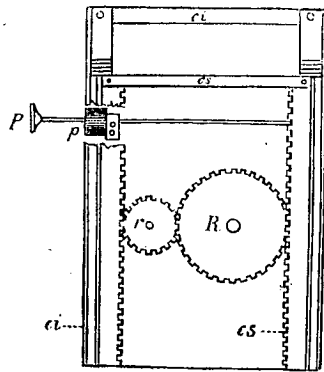
Figure 24. Chariot du fusil photographique.
