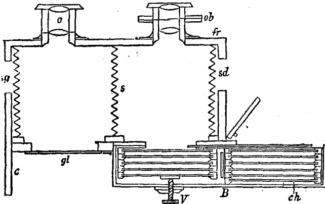
Figure 23. — Fusil photographique du docteur Fol.
