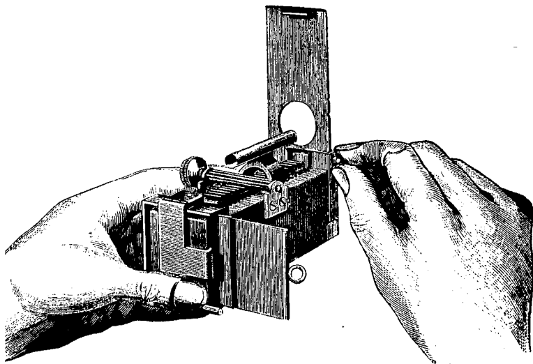
Figure 28. — Chambre de Marion.
