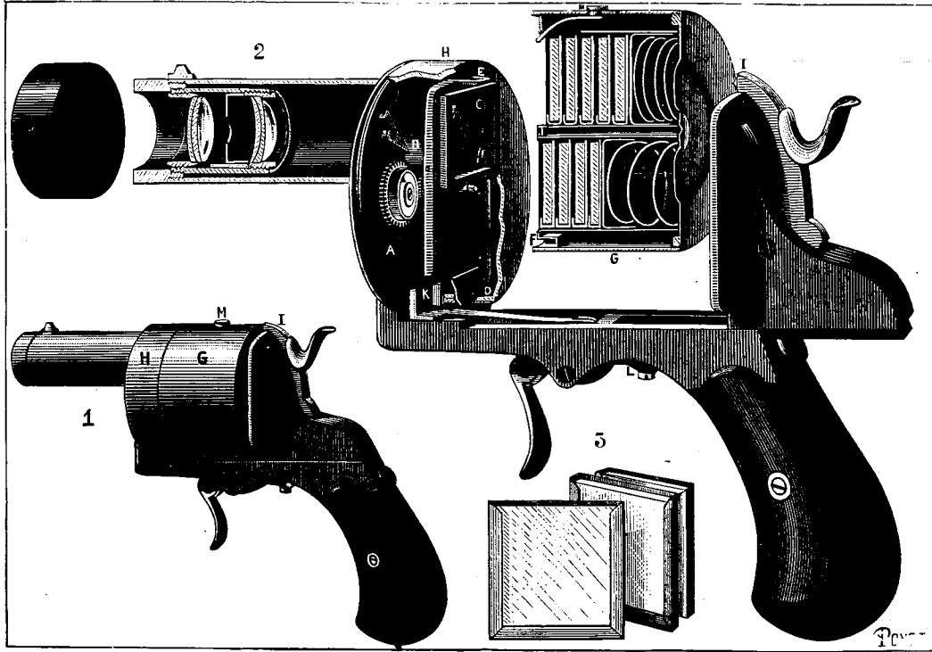
Figure 22. - Revolver photographique de M. Enjalbert.
