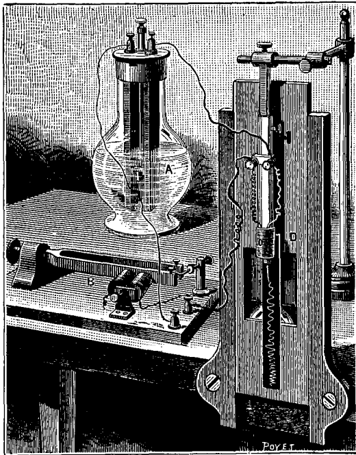
Figure 19. — Chronographe pour déterminer la vitesse d'un obturateur.
