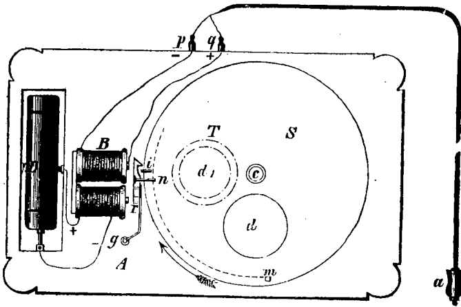
Figure 16. -- Obturateurs à disque rotatif avec déclenchement électrique.
