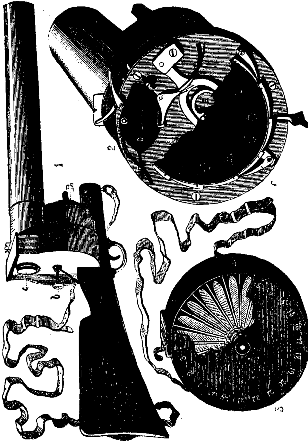
Figure 145. — Mécanisme du fusil photographique de Marey. — 1. Vue d'ensemble. — 2. Vue de l'obturateur et du disque percé-plaques. — 3. Boîte à escamoter pour vingt cinq glaces.
