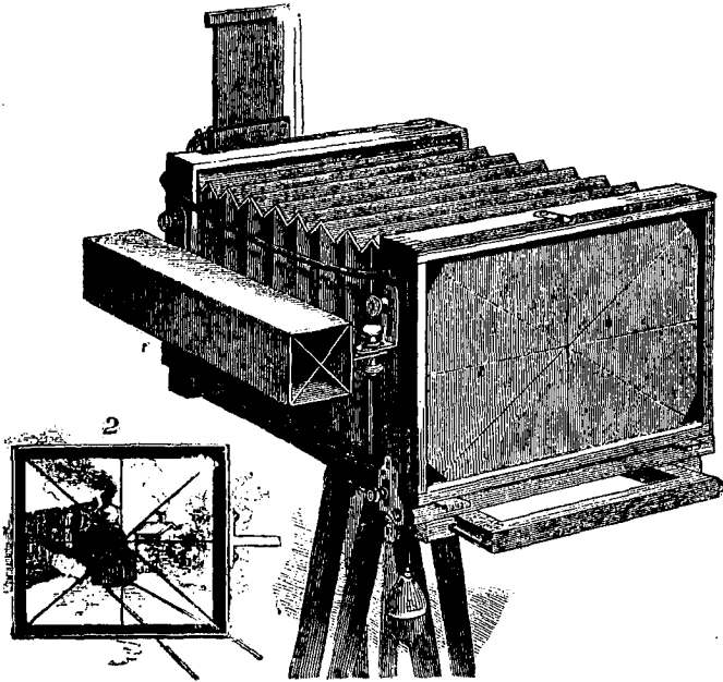
Figure 31. — Chambre noire munie d'un iconomètre ou chercheur.
