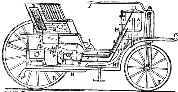
Figure 4. — Voiture RAVEL, 1868 (Fr. A.).
