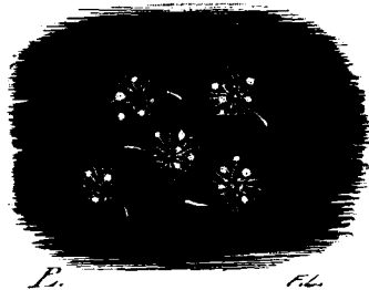
Fig. 81. — Noctiluques.
