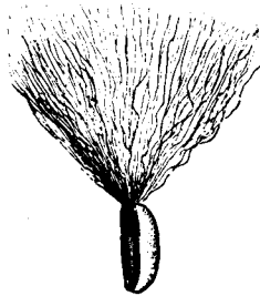
Fig. 51. — Graine d'Épilobe.
