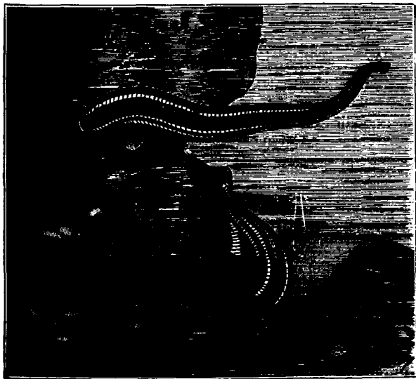
Fig. 99. — La Sangsue.
