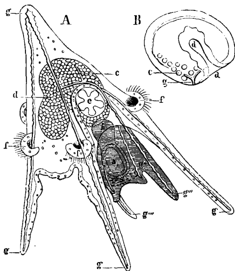
Fig. 91. — Larves d'Oursins.
