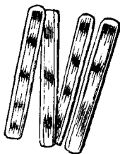
Fig. 19. — Diatomées.
