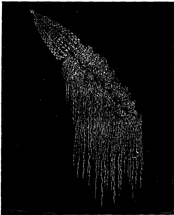
Fig. 89. — Un Siphonophore.
