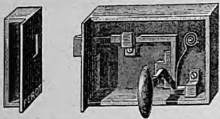
SEERRURE APPELÉE REC DE CANE. — C'est la serrure la plus simple. Il suffit, pour la fermer, de pousser la porte; le ressort, qu'on voit à droite, la maintient fermée.
