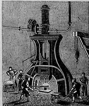
LE MARTEAU-PILON À VAPEUR. — On emploie maintenant, pour la construction des ponts en fer ou des grandes machines, des pièces de métal tellement grosses, qu'aucun marteau mû par une main d'homme ne pourrait les façonner. Pour les forger, on a inventé l'énorme marteau-pilon que la vapeur met en mouvement et qui peut frapper depuis deux cents jusqu'à cinq cents coups par minute.
