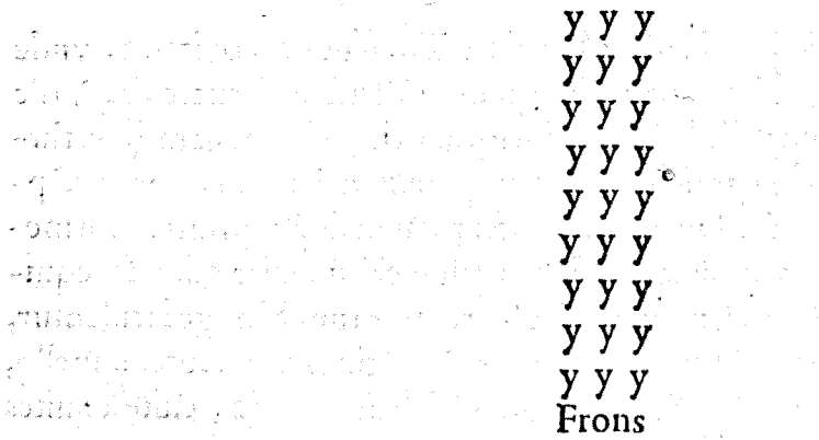
Phalanx transuersa.
